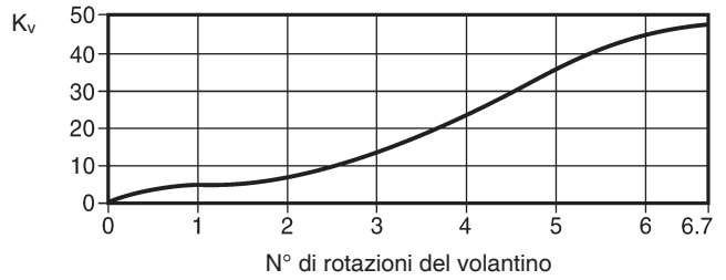
BSAT - DN80
