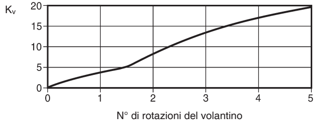
BSAT - DN50
